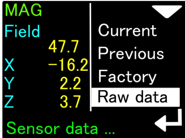
Magnetometer-Rohdaten
